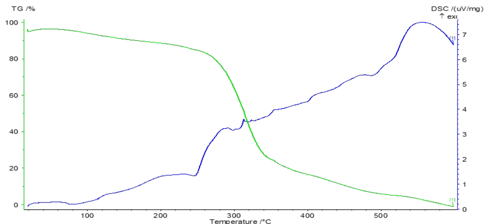
Рисунок 2 – Термогравиметрический анализ анионита на основе А-ЭХГ-ПЭПА.
