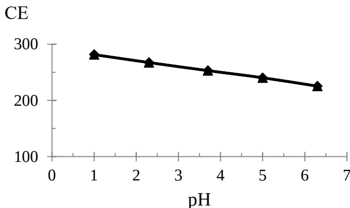
Рисунок 4 – Зависимость сорбции ионов \text{Sr}^{2+} анионитом А–ЭХГ–ПЭПА от кислотности раствора \text{SrCl}_2 . c_{\text{Sr}} = 2,015 \text{ г} \cdot \text{л}^{-1} , время контакта 7 сут.
