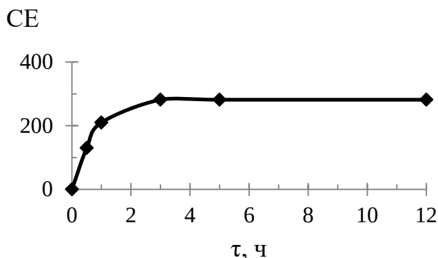
Рисунок 5 – Зависимость сорбции ионов стронция (II) анионитом А–ЭХГ–ПЭПА от продолжительности его контакта с раствором \text{SrCl}_2 ( c_{\text{Sr}} = 2,015 \text{ г} \cdot \text{л}^{-1} , pH = 1,0)
